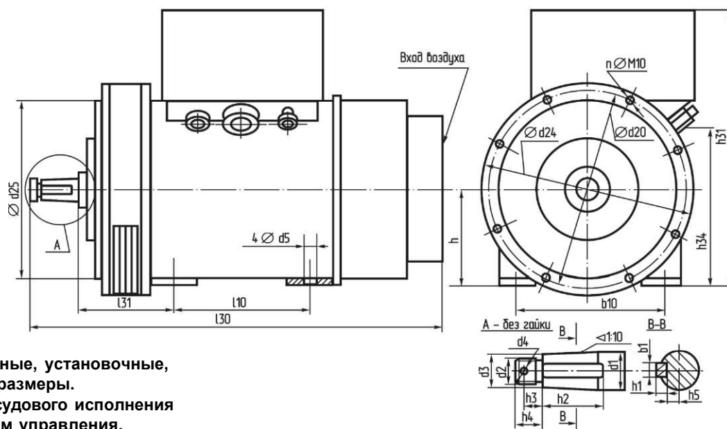
Рисунок №8. Габаритные, установочные, присоединительные размеры. Генератор серии БГ судового исполнения.
