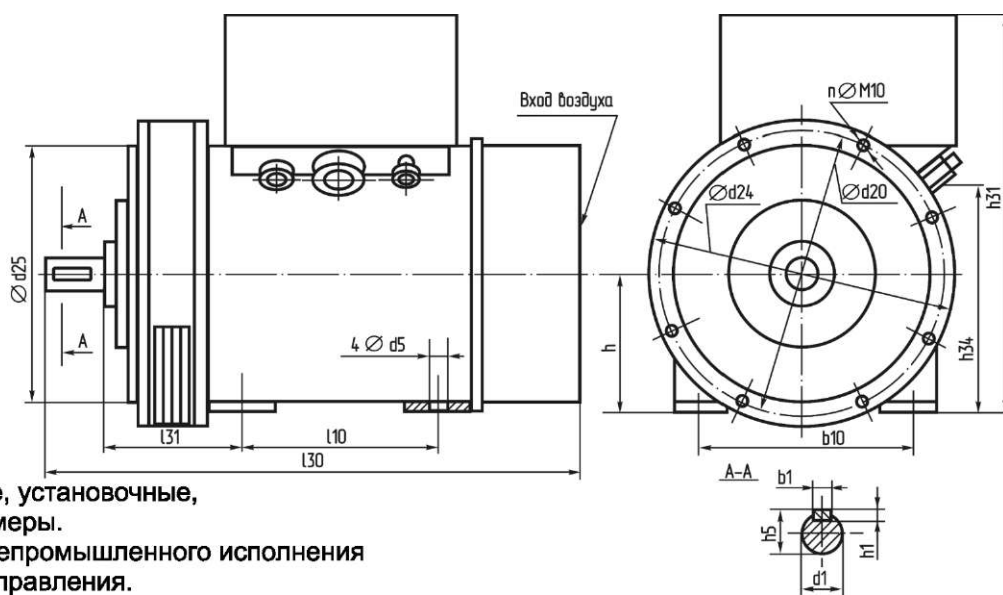
Рисунок №5. Габаритные, установочные, присоединительные размеры. Генератор серии БГ общепромышленного исполнения.
