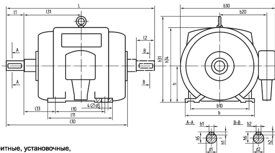
Рисунок №21. Габаритные, установочные, присоединительные размеры. Высоковольтные электродвигатели серии AO4. IM 1001, IM 1002.
