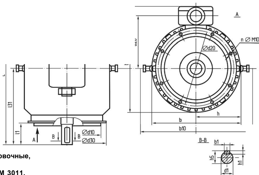
Рисунок №27. Габаритные, установочные, присоединительные размеры. Электродвигатели серии А02-9. IM 2001, IM 2002.
