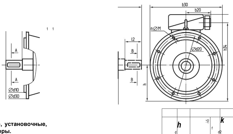
Рисунок №36. Габаритные, установочные, присоединительные размеры. Электродвигатели серии 4АЛ. IM 1001, IM 1002.
