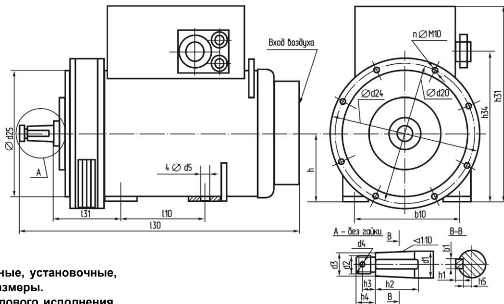
Рисунок №9. Габаритные, установочные, присоединительные размеры. Генератор серии БГ судового исполнения со встроенным блоком управления.
