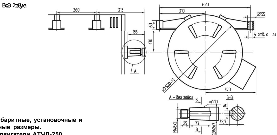
Рисунок №37. Габаритные, установочные, присоединительные размеры. Электродвигатели серии 4АЛ. IM 3001, IM 3002.
