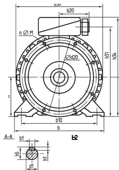
Рисунок №17. Габаритные, установочные, присоединительные размеры. Электродвигатели серии 5AM. 5AM-200, 5AM-250. IM 2001, IM 2002.
