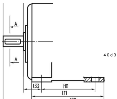
Рисунок №33. Габаритные, установочные, присоединительные размеры. Крановые электродвигатели серии АИК. IM 1001, IM 1002.
