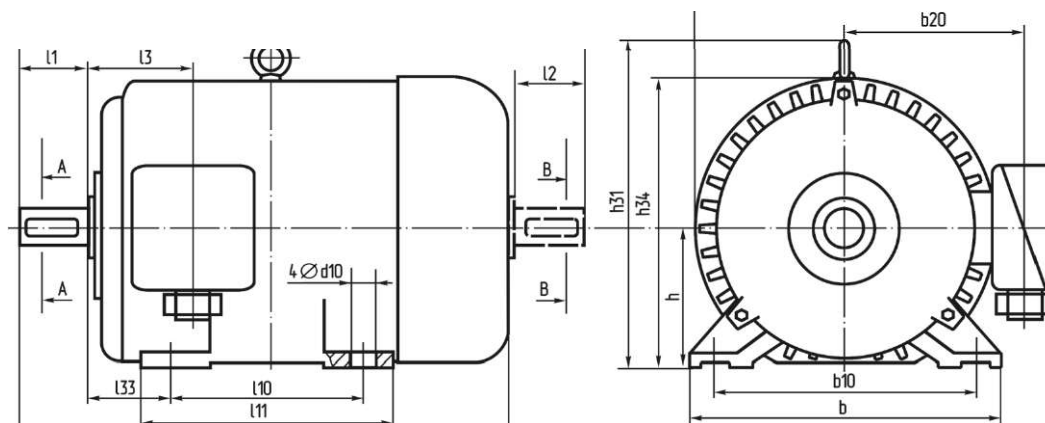
Рисунок №29. Габаритные, установочные, присоединительные размеры. Многоскоростные электродвигатели серии А02-9. IM 1001, IM 1002.
