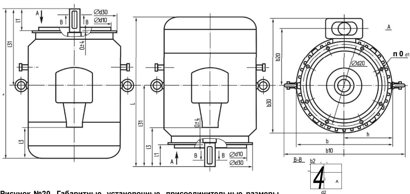
Рисунок №20. Габаритные, установочные, присоединительные размеры. Низковольтные и высоковольтные электродвигатели серии A04. IM3011, IM 3031.
