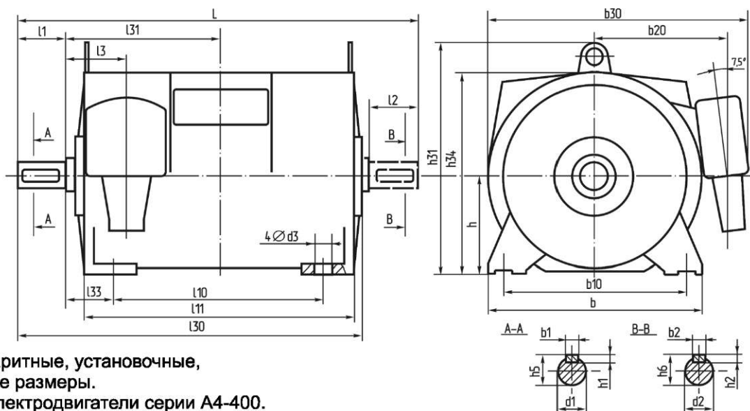
Рисунок №22. Габаритные, установочные, присоединительные размеры. Высоковольтные электродвигатели серии A4-355. IM 1001, IM 1002.
