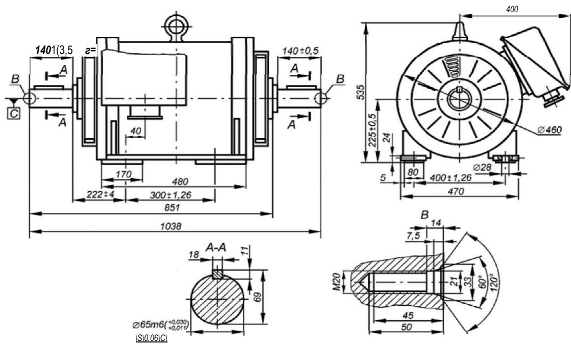
Габаритные, установочные и присоединительные размеры двигателя АНЭ22514УХЛ2. Монтажное исполнение IM 1001, IM 1002.
