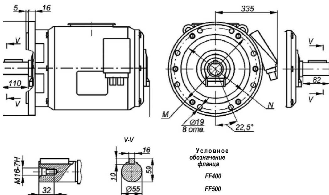
Габаритные, установочные и присоединительные размеры двигателя 5АН200М...НЛБ. Монтажное исполнение ИМ3001, ИМ3002
