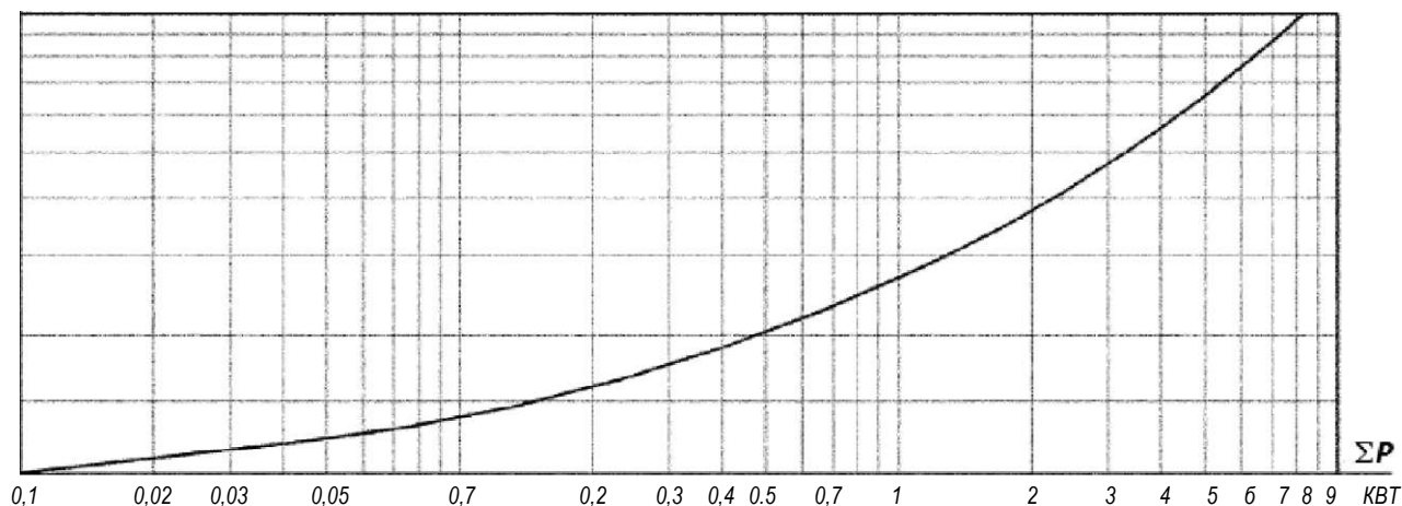
Рисунок 5. Зависимость расхода воздуха Q, необходимого для охлаждения встраиваемых двигателей, от суммарных потерь \Sigma P
