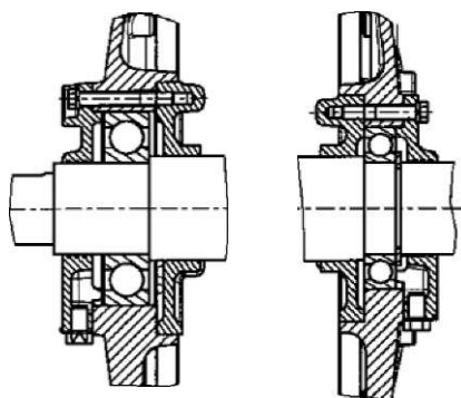
Рисунок 14.3 для двигателей габаритов 200 - 280 мм
