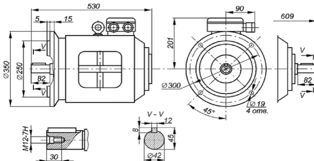
Габаритные, установочные и присоединительные размеры двигателей 5АН 160S...НН5. Монтажное исполнение IM3001, IM3002
