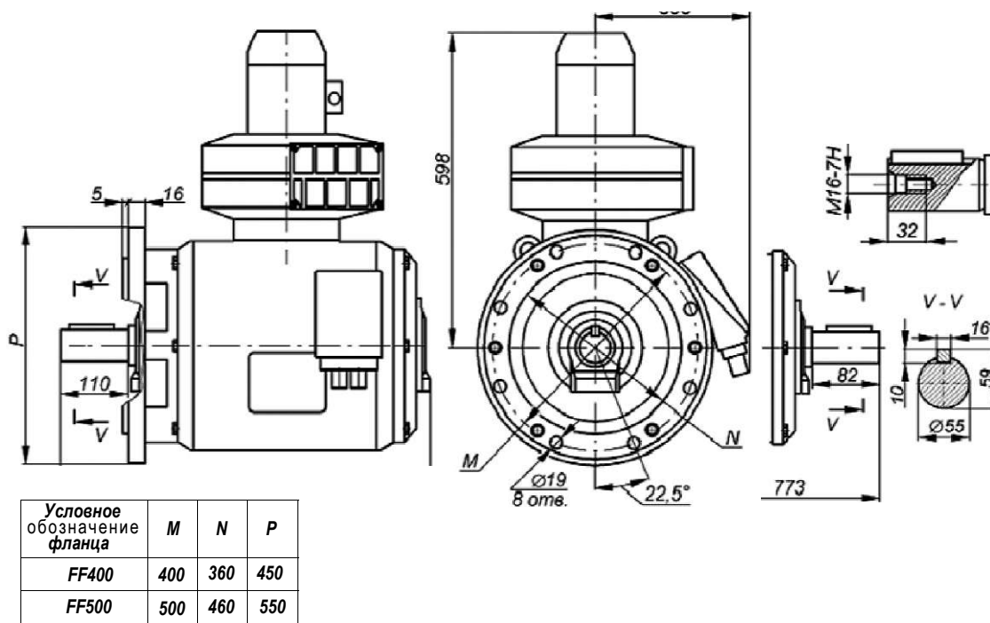
Габаритные, установочные и присоединительные размеры двигателя 5АФ200М...НЛБ. Монтажное исполнение ИМ3001, ИМ3002
