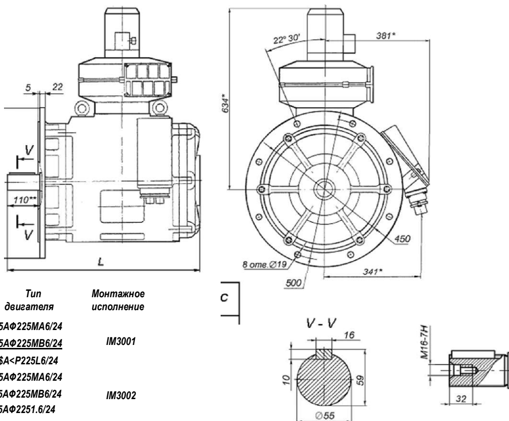
Габаритные, установочные и присоединительные размеры двигателя 5АФ225...НЛБ. Монтажное исполнение IM3001, IM3002
