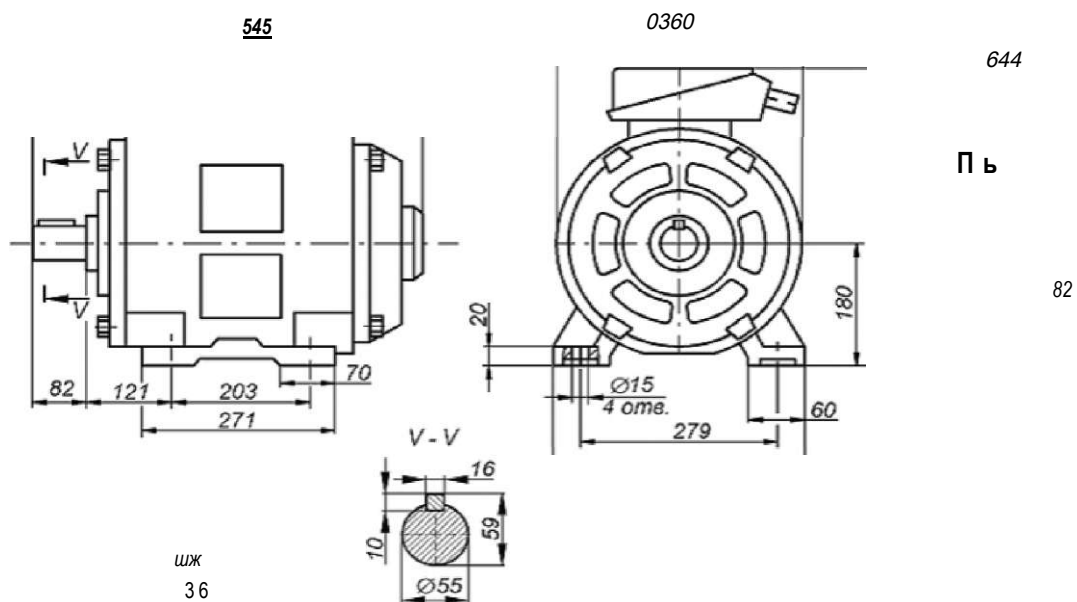
Габаритные, установочные и присоединительные размеры двигателя 5АН180S6/24Н/1В. Монтажное исполнение IM1001, IM1002
