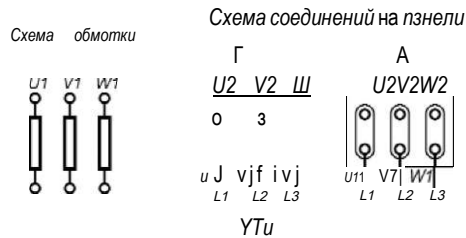
Рисунок 7.1 для односкоростных двигателей с соединением в звезду (Y), в треугольник (A) или переключаемых: звезда - треугольник (Y/A).
